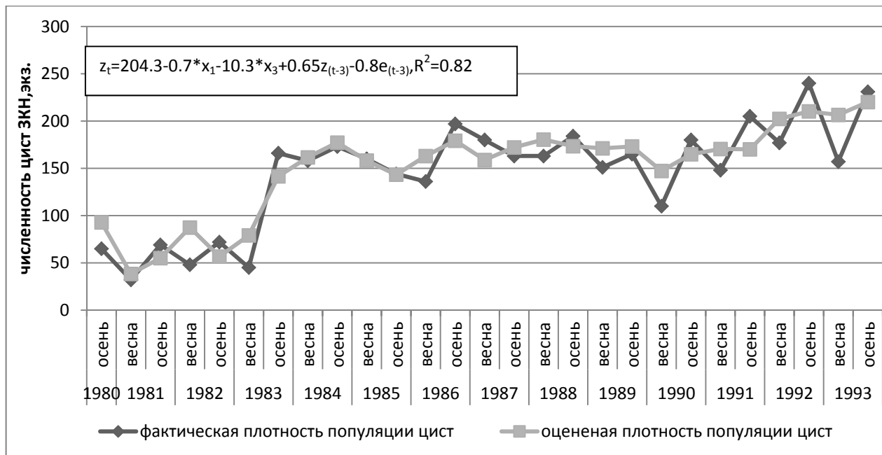
Рис.7. Фактическая численность цист ЗКН, численность смоделированная с включением данных о динамике популяции, температуры почвы марта, уровня осадков мая.
