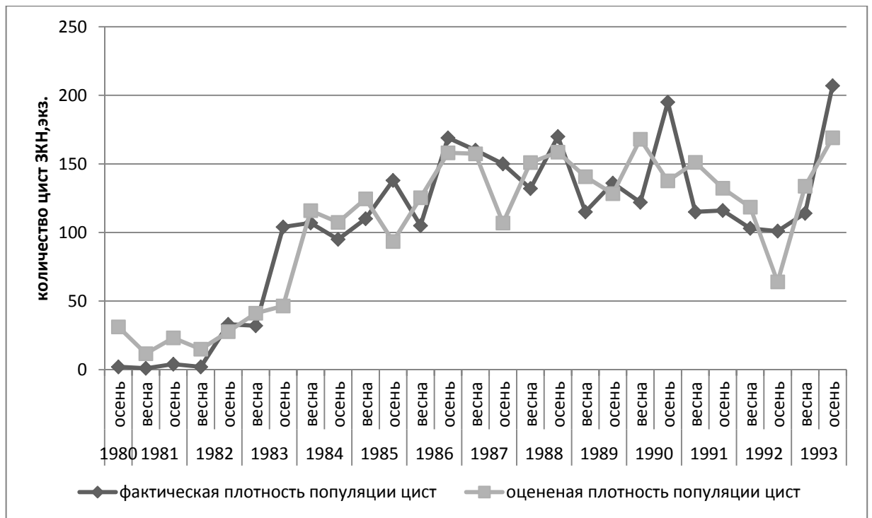
Рис. 3. Фактическая численность цист ЗКН, численность смоделированная с включением данных о динамике популяции и температуре почвы сентября
