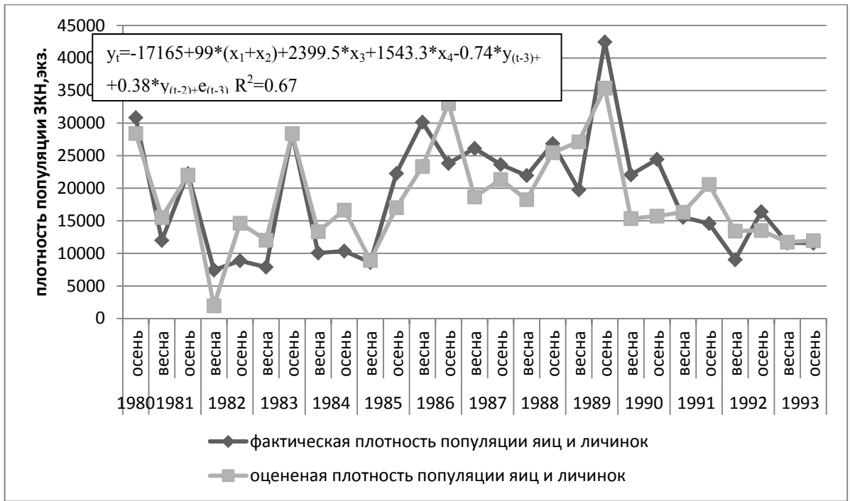
Рис. 4. Фактическая ПП ЗКН, плотность популяции смоделированная с включением данных о динамике популяции, температуры почвы марта и июня, уровня осадков мая и июня
