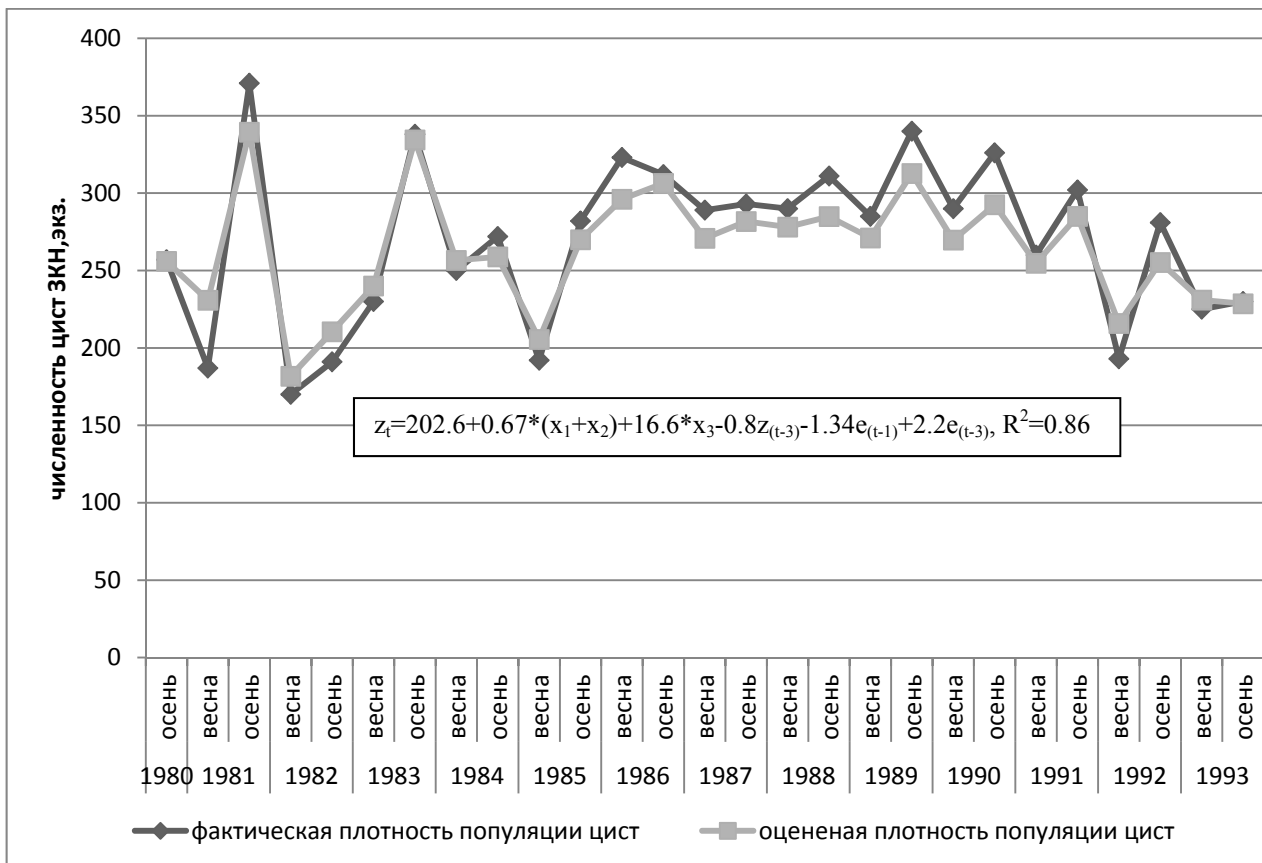
Рис. 5. Фактическая численность цист ЗКН, численность смоделированная с включением данных о динамике популяции, температуры почвы марта, уровня осадков мая и июня 3. Модель, объясняющая динамику плотности популяции ЗКН в почве участка с низким уровнем плодородия на 72%:
